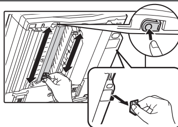
Podávací válec
