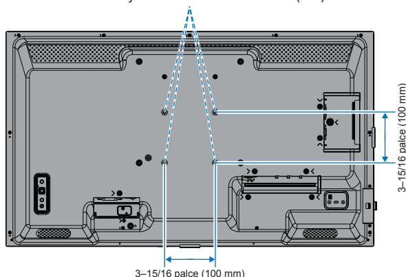
Montážní vybavení standardu VESA (M4)
